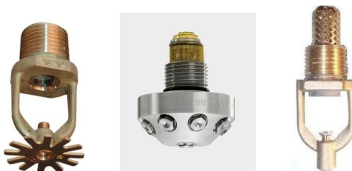
Рисунок 5 - Дренчерный ороситель
